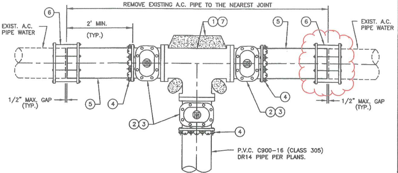
PLAN N.T.S.
